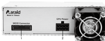
圖4. ARAID M6 後視圖
